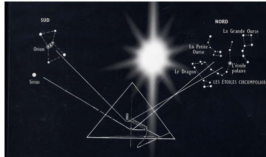
Situation du ciel au moment du Zep-Tepi (11540 Av JC)
